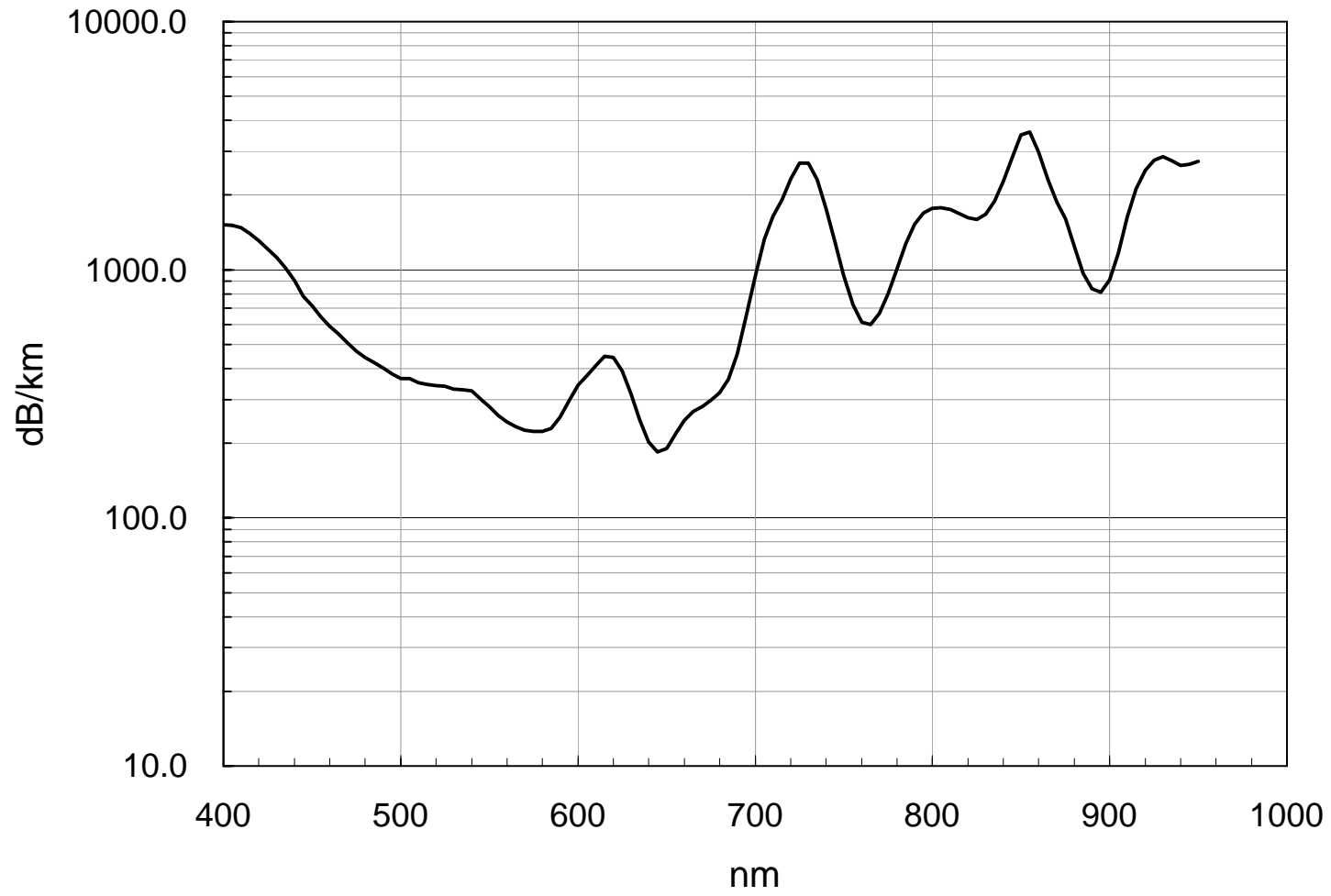
Spectral Attenuation (OM-Giga)
