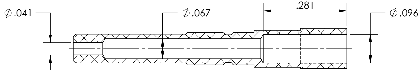
SECTION A-A SCALE 5 : 1
